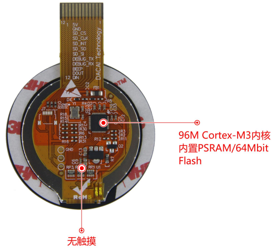
图 1-2 硬件配置图
